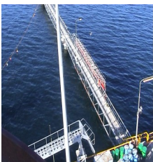
Σύστημα Κλειστού κυκλώματος τηλεόρασης σε πλατφόρμα Φορτοεκφόρτωσης καυσίμων στην Ελευσίνα (Μεγαρίχελ IP κάμερες, Marine & ATEX exd grade)
