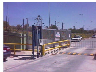
Σύστημα Ελέγχου Πρόσβασης και Κλειστού κυκλώματος σε γεμιστήρια Καυσίμων στην Κρήτη (τουρνικέ, αυτόματες μπάρες, Ενδείξεις)
