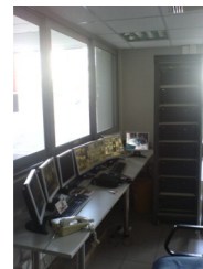
Σύστημα Κλειστού Κυκλώματος σε εμπορικό κέντρο αναφυχής (225 κάμερες—3 control room) στην Αθήνα
